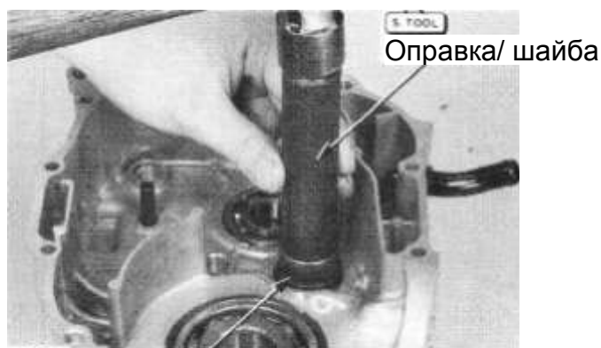
Оправка/ шайба
