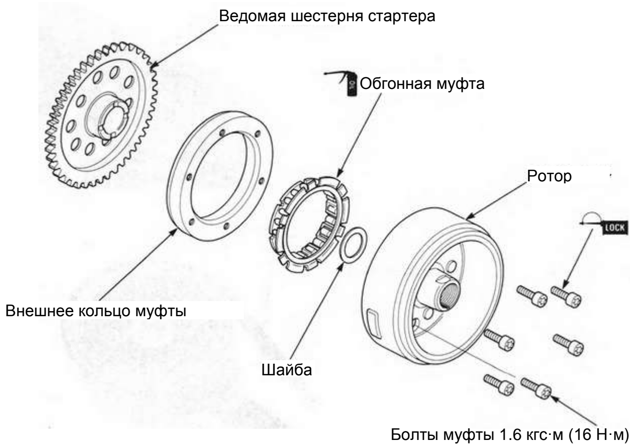
Муфта
