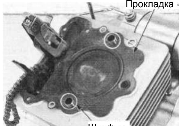
Штифты
