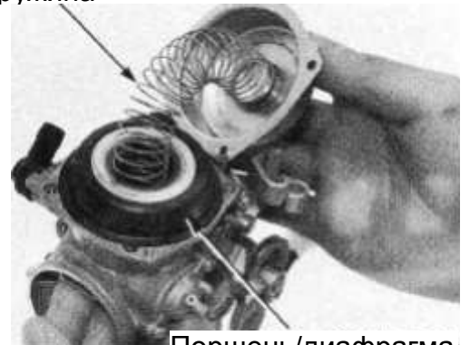
Поршень/диафрагма
