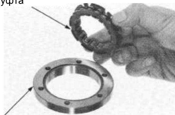
Внешнее кольцо
