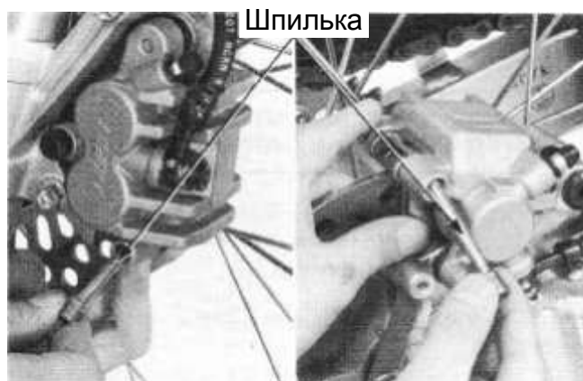
Колодки
