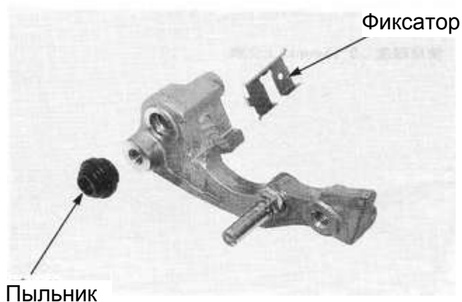
Суппорт
