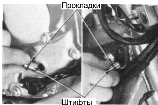
Маслопроводы
