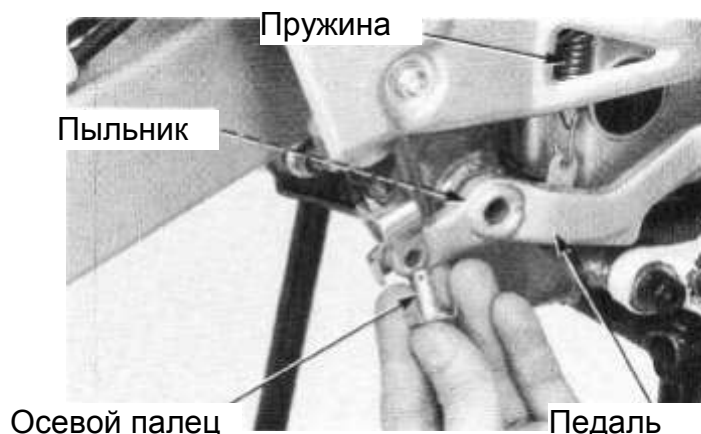
Педаль
