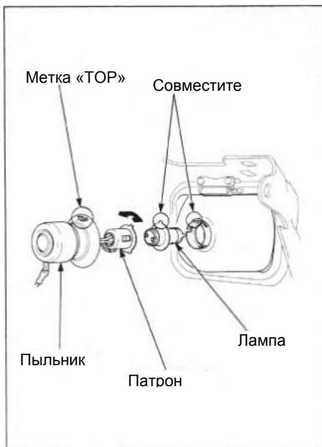
Пыльник
