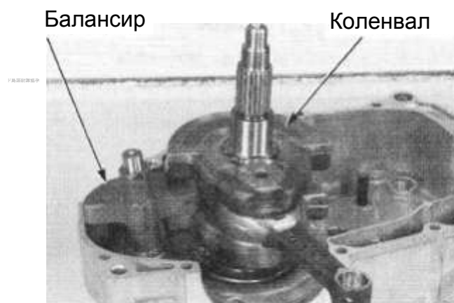
Балансир
