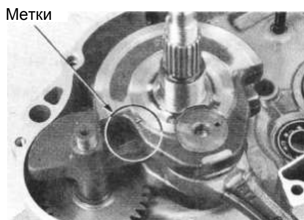
Валы КПП
