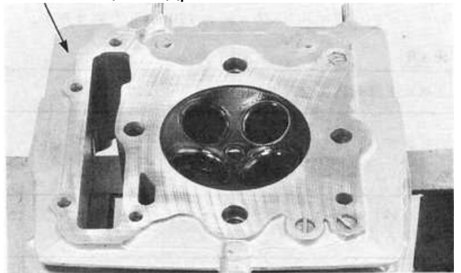
Головка цилиндра
